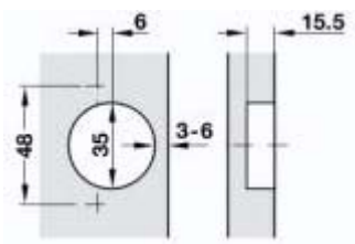
чрез винтове 48/6
